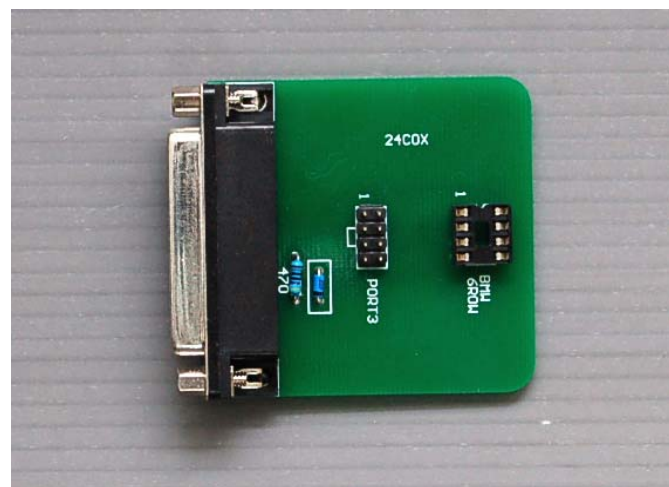
eprom-24xx
