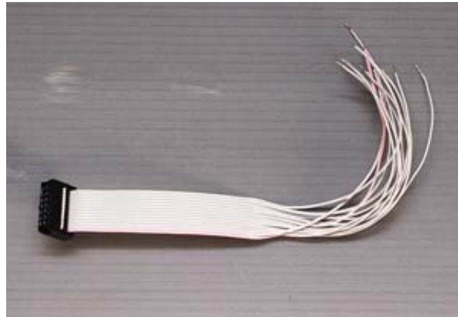
eprom-14pin
