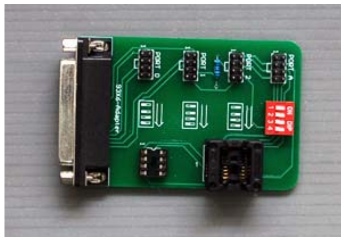
eprom-93xx
